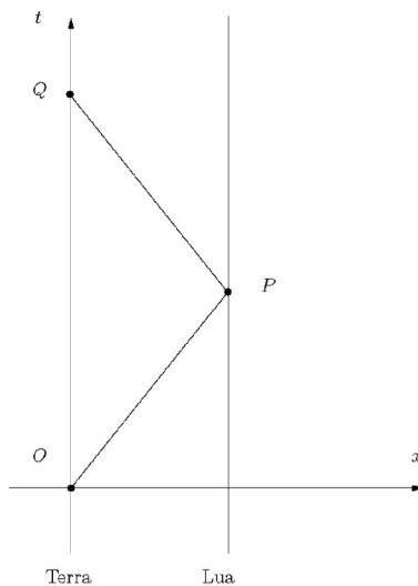
Figura 2 - Paradoxo dos gémeos
