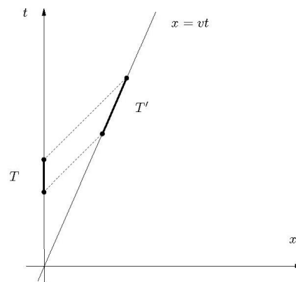
Figura 3 - Efeito de Doppler
